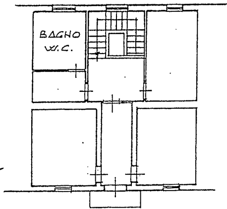
PIANO PRIMO H. 2.80
